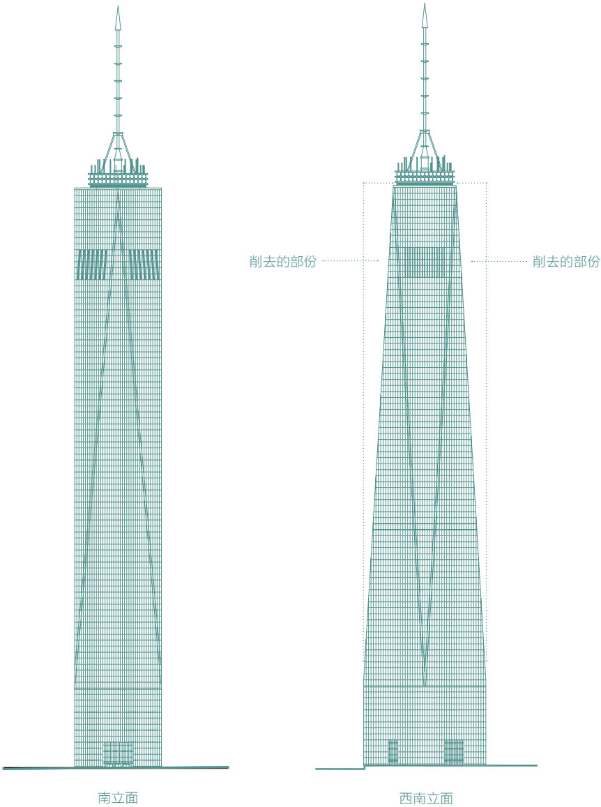
世界貿易中心一號大樓結構圖
