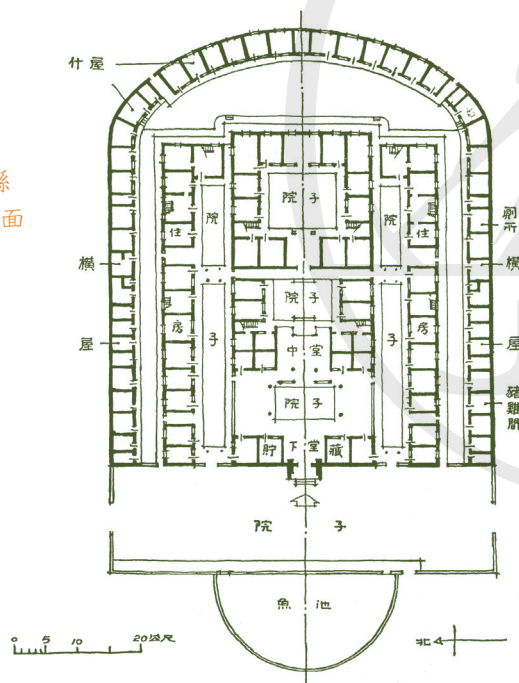
圖 115 福建省永定縣客家 住宅底層平面 (中國建築研究室調查)
