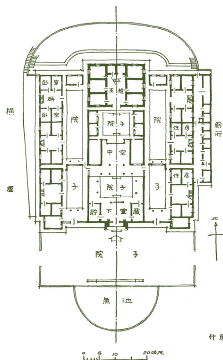
圖 114 福建省永定縣 客家住宅大夫第底層平面 (中國建築研究室調查)
