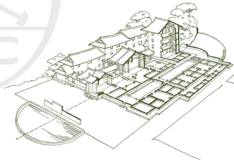
圖 117 福建省永定縣客家住宅大夫第剖視 (中國建築研究室調查)
